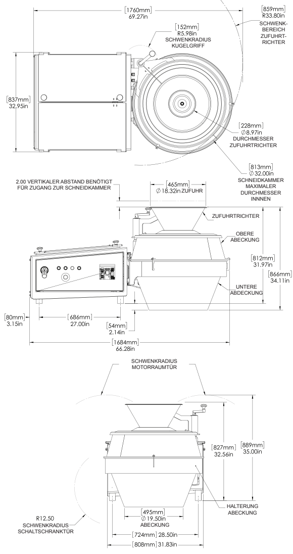
Schneidkammer 32"
