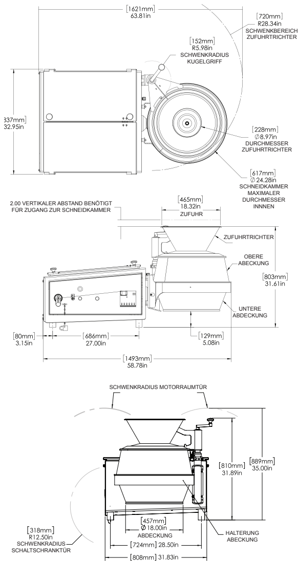
Schneidkammer 24"
