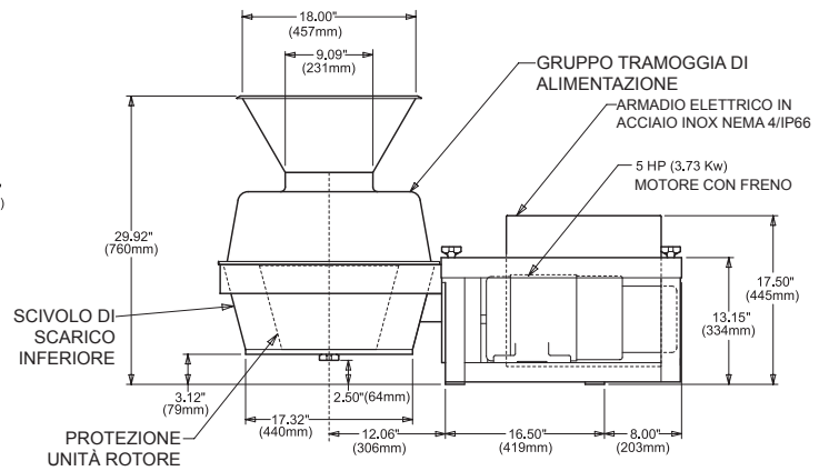
Modello CC-D provvisto di motore da 5 CV
