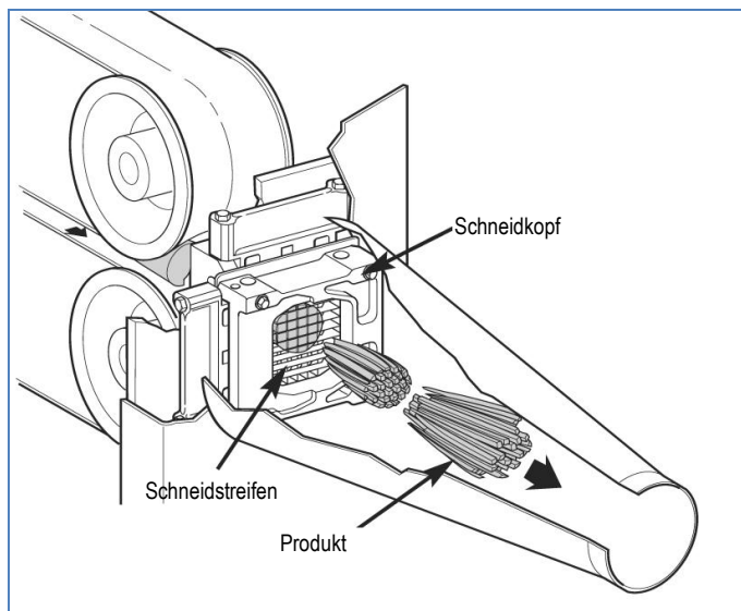
MODELL VSC MIT VELOCICUT® SCHNEIDKOPF
